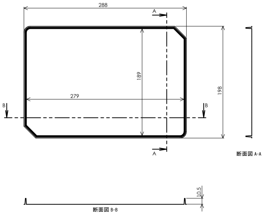
断面図 B-B
